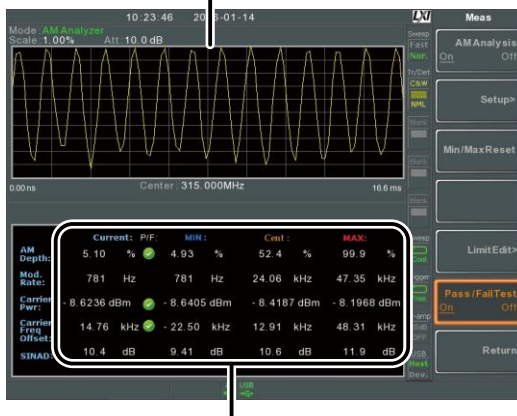
AM変調の測定値
