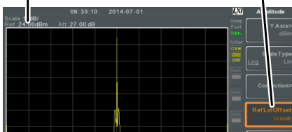
リファレンスレベル設定後 (オフセット: 10dB)
