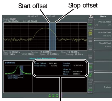
位相ジッタ測定
